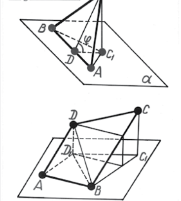
163. Площадь ортогональной проекции треугольника Теорема 18.1.
