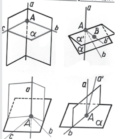
150. Расстояние между скрещивающимися прямыми
