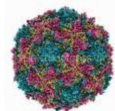
Вирус полиомиелита имеет форму додекаэдра
