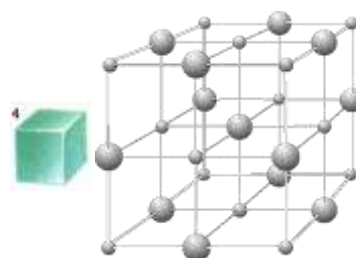
Куб- монокристалл поваренной соли
