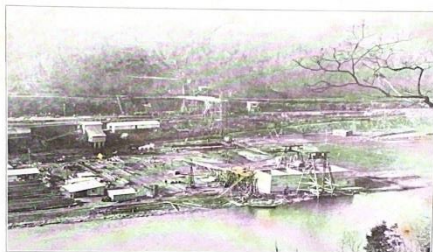
Reichsautobahn Göttingen-Kassel Bau der Werrebrücke bei Hann. Münden (Pfeiler und Widerlager — a. T. Lohdrückgründung) Bauweise für Pfeiler
